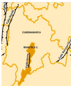
Fuente: Fallas geológicas activas cercanas a la ciudad de Bogotá (adaptado de GEM & SGC, 2017)
